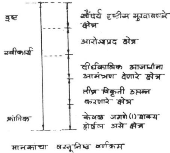
आकृती ५.२ : मानकांचा वस्तुनिष्ठ वर्णक्रम
