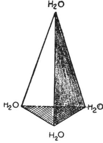
आकृती ३.३ : चतुष्फलकाच्या टोकाशी जोडलेले पाण्याचे रेणू.
