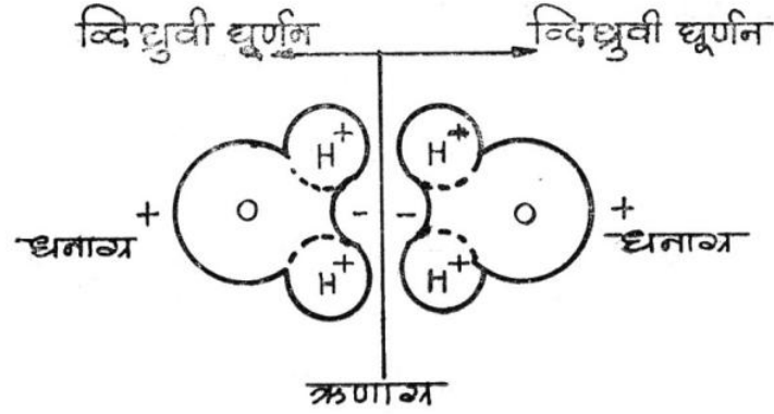
आकृती ३.४ : पाण्याचे द्विध्रुवी घूर्णन.
