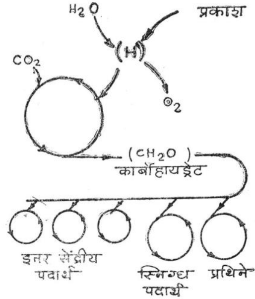
आकृती २.२ : प्रकाशसंश्लेषी क्रियांचा समूह
