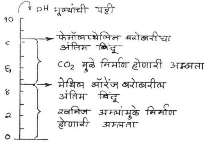
आकृती ७.२ : महत्त्वपूर्ण अम्लतांचे विविध प्रकार व त्यांचे pH मूल्यांशी असलेले संबंध
