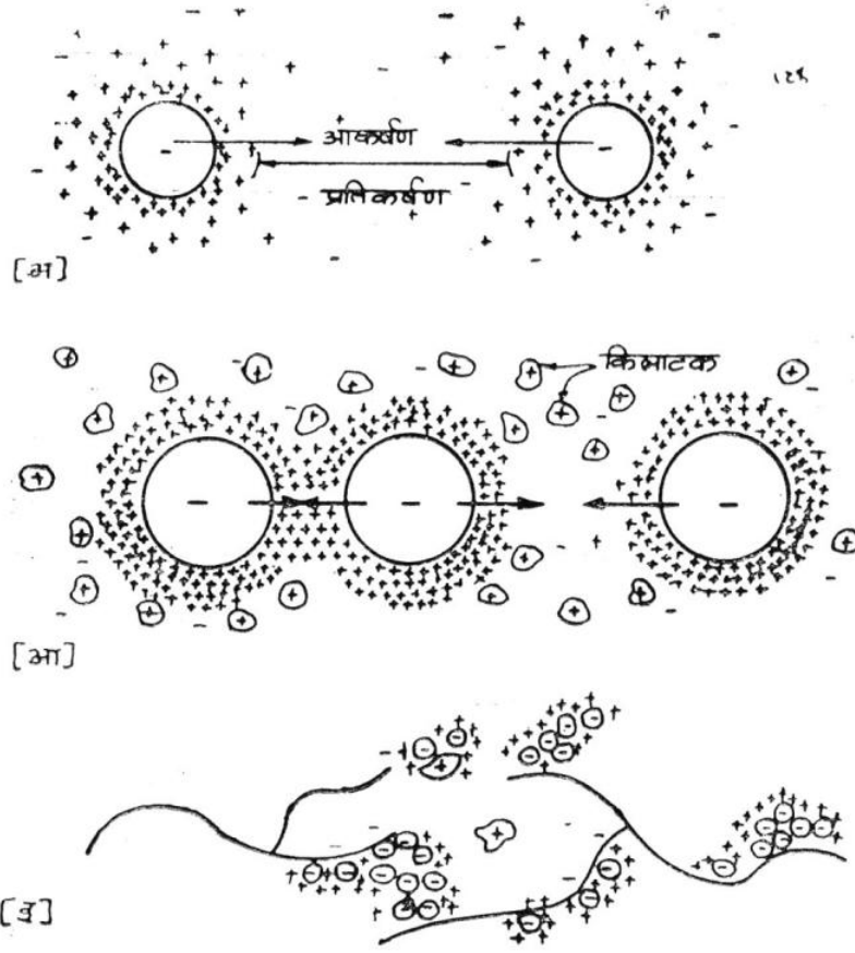
आकृती ९.१ कलीले आणि किलाटक यांच्यामधील कार्यप्रदर्शी अभिक्रिया.
