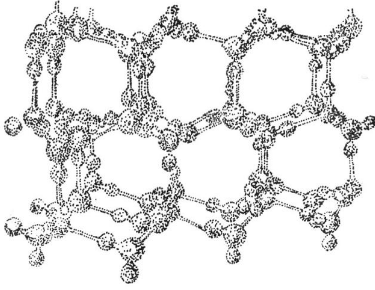
बर्फाच्या खड्डा
