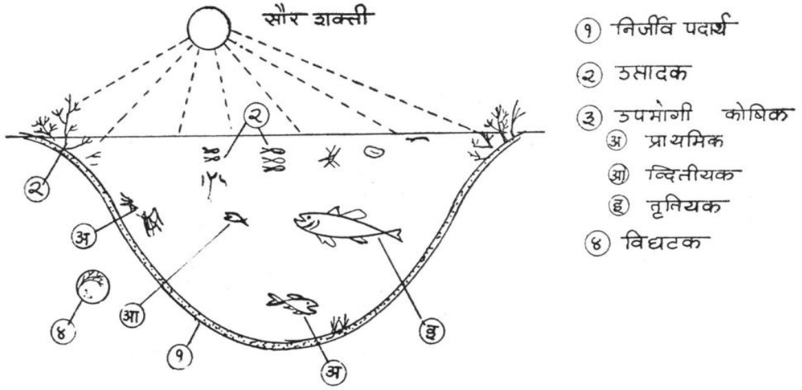
आकृती ६.१ : नैसर्गिक परिस्थितीत आढळणारी अन्नसाखळी
