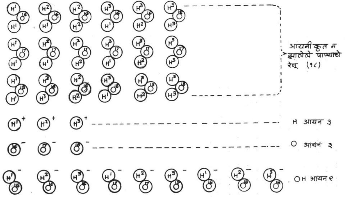
आकृती ४.१ : पाणी म्हणजे, १८ रेणू आणि १५ निरनिराळे आयन यांनी मिळून झालेले एक रासायनिक मिश्रण.
