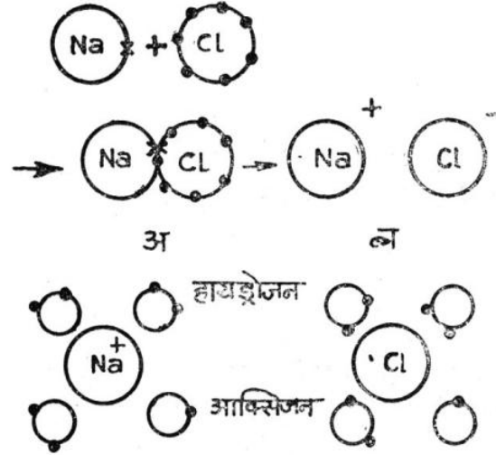
आकृती ३.५ : सोडियम क्लोराईडचे पाण्यात विलयन.
