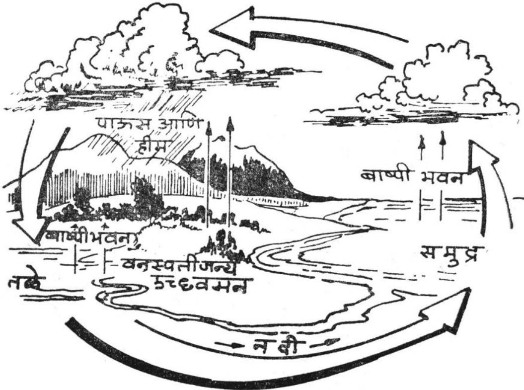
आकृती १-१ : जलचक्र
